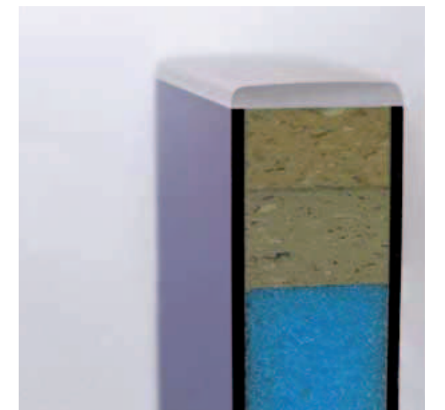
Nassfeste Türblätter Stumpf einschlagend oder überfält, auch für vorhandene Standardzargen verwendbar. Hartschaumkern mit verstärktem Randbereich, beidseitig mit 3 Millimeter HPL-Compact belegt, umlaufend fugenlos angegossene, schlagzähe PUR-Kante.
